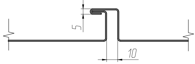
Соединение двух смежных кассет
