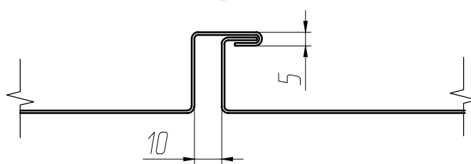
Соединение двух смежных кассет
